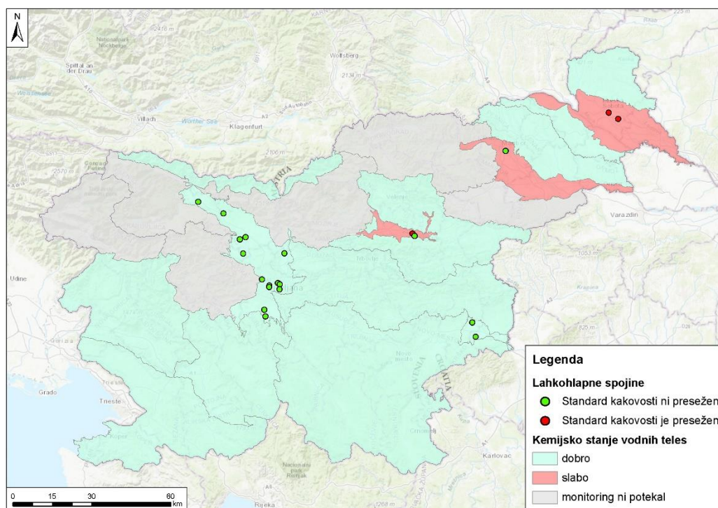
Slika 7: Vsebnost lahkohlapnih halogeniranih ogljikovodikov v podzemni vodi v letu 2019 (rezultati monitoringa ARSO; Dobnikar Tehovnik et al., 2020).
