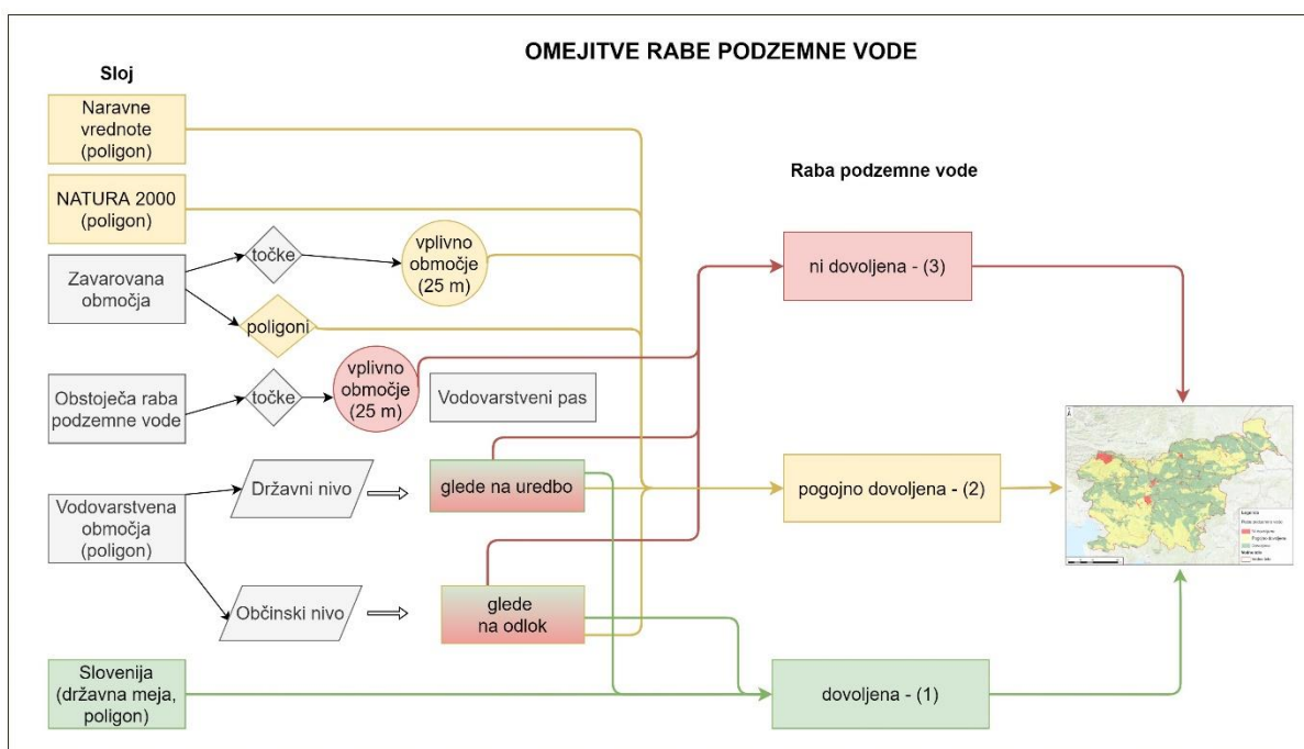
Slika 35: Diagram postopka določitve omejitev rabe podzemne vode za namene akvakulture.
