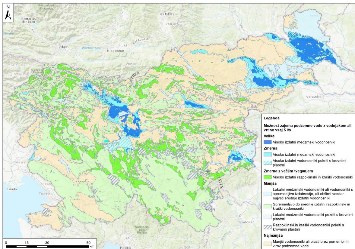
Slika 29: Možnost zajema 5 l/s podzemne vode z vrtino/vodnjakom.
