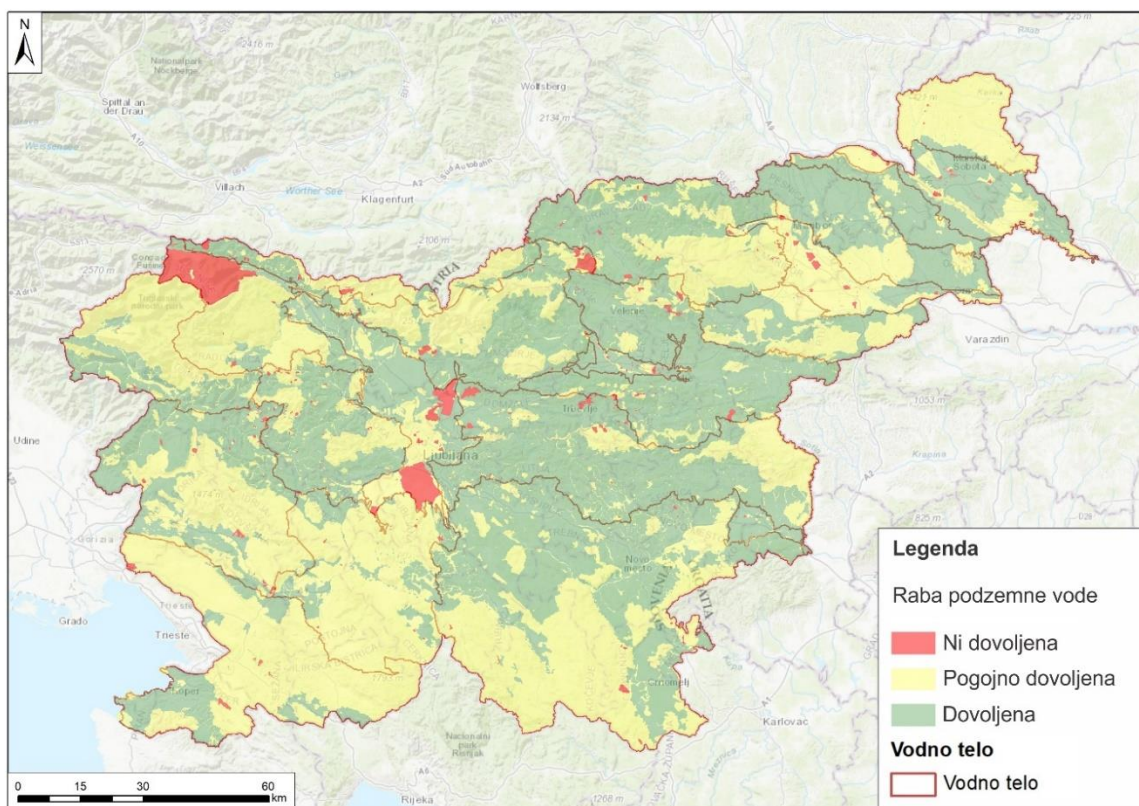
Slika 38: Možnost rabe podzemne vode za namene akvakulture.
