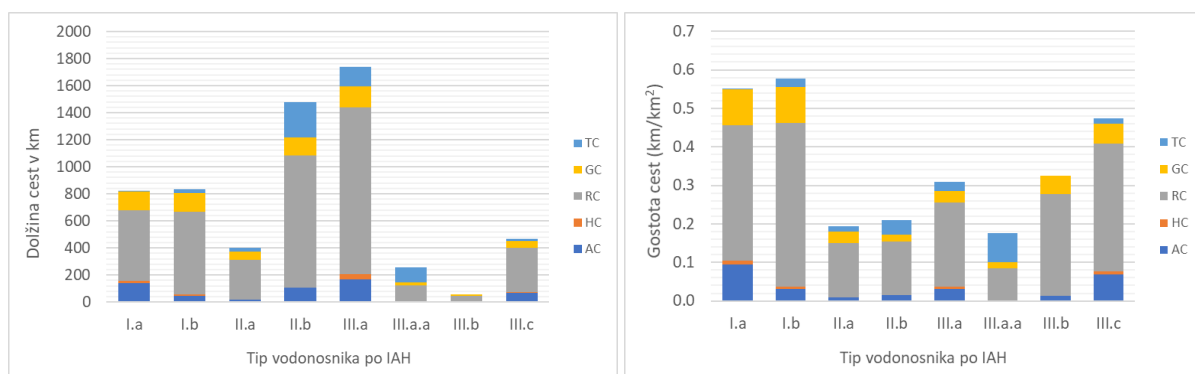
Slika 19: Dolžina državnih cest in gostota državnih cest po tipih vodonosnikov po IAH, kjer izvajajo štetje prometa (vir podatkov: Direkcija RS za infrastrukturo, 2020).
