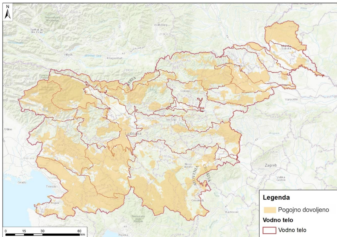
Slika 36: Omejitve rabe podzemne vode za namene akvakulture na naravovarstveno pomembnih območjih.
