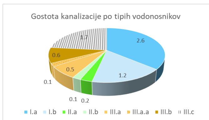
Slika 17: Gostota kanalizacijskega omrežja na površino posameznega tipa vodonosnikov po IAH (km/km²).
